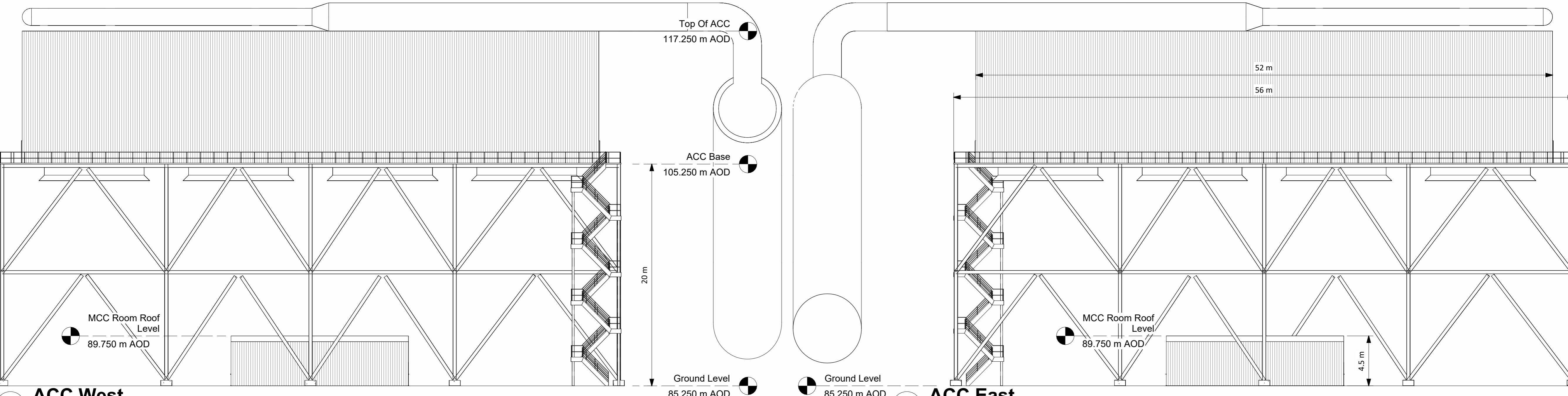
3 ACC West 1 : 200
